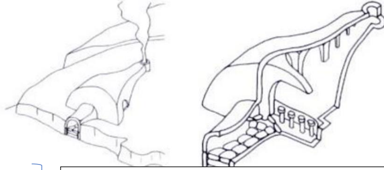
Şekil 1.1. Geleneksel Anagama Seramik Fırınının tasarımı ve çizimi
